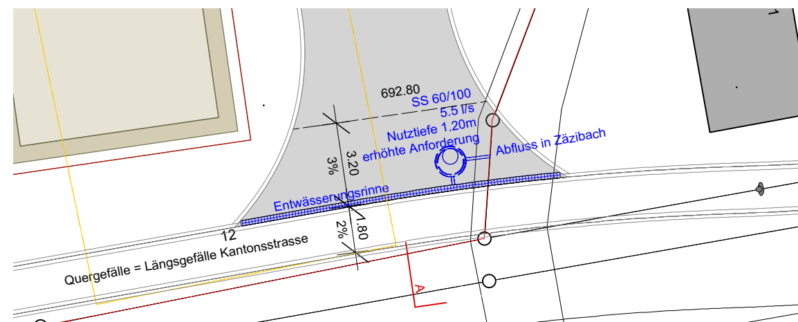
Entwässerung 1:200
